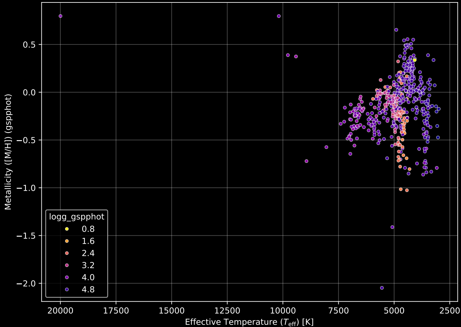
APOGEE DR17 Field: [N752_btx] Stellar Population Parameters (n= 522)
